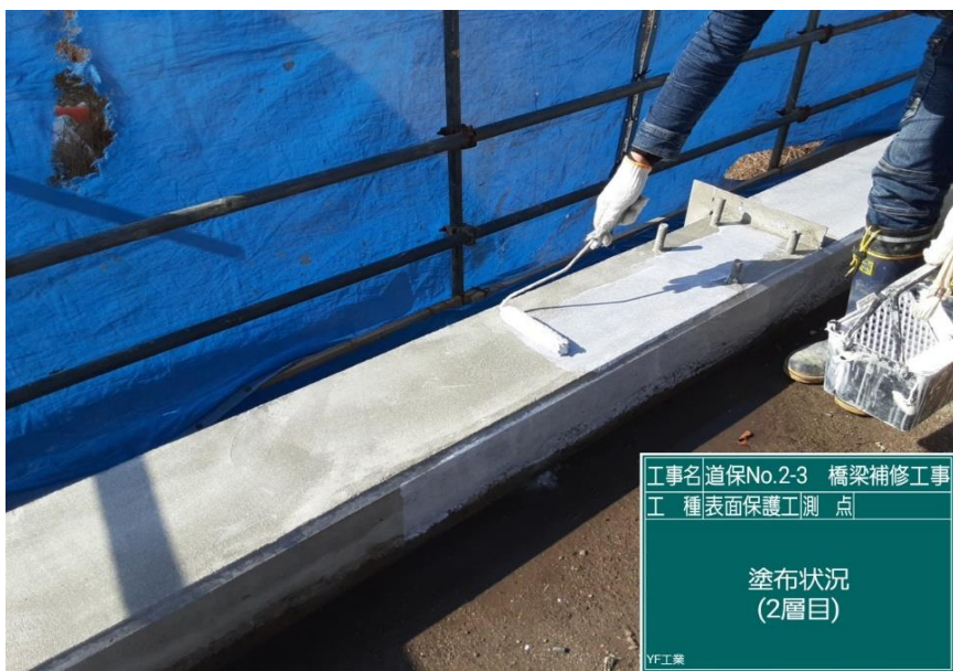
施工状況 地覆部の断面修復後、中性化や塩害等の劣化抑制のため、浸透性のある保護材の塗布状況
